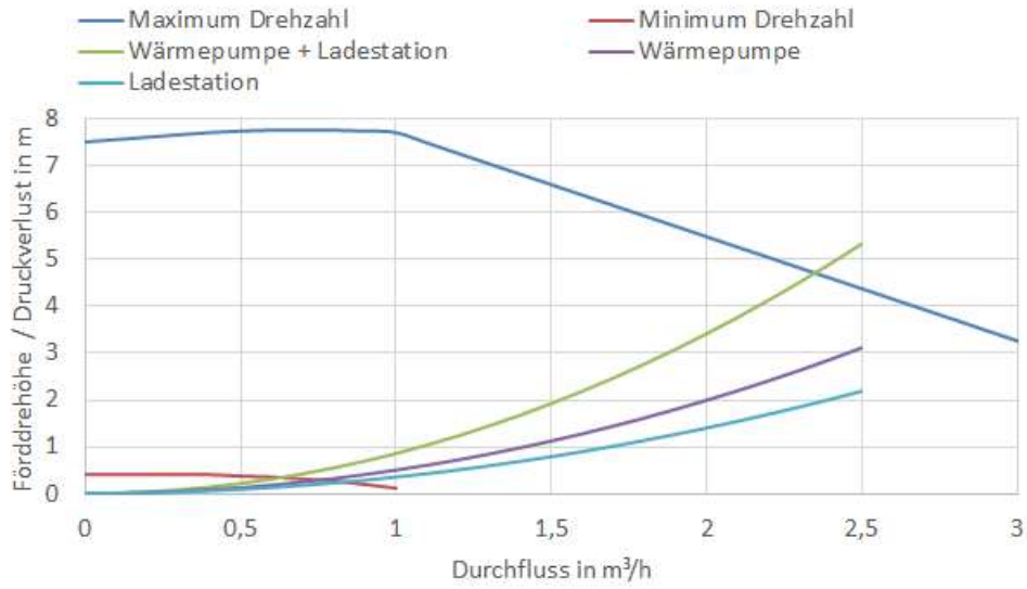
Abbildung 35: Pumpenkennlinie Grundfoss UPM3L 75/180 und Anlagenkennlinie
