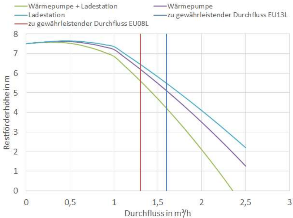
Abbildung 36: Restförderhöhe
