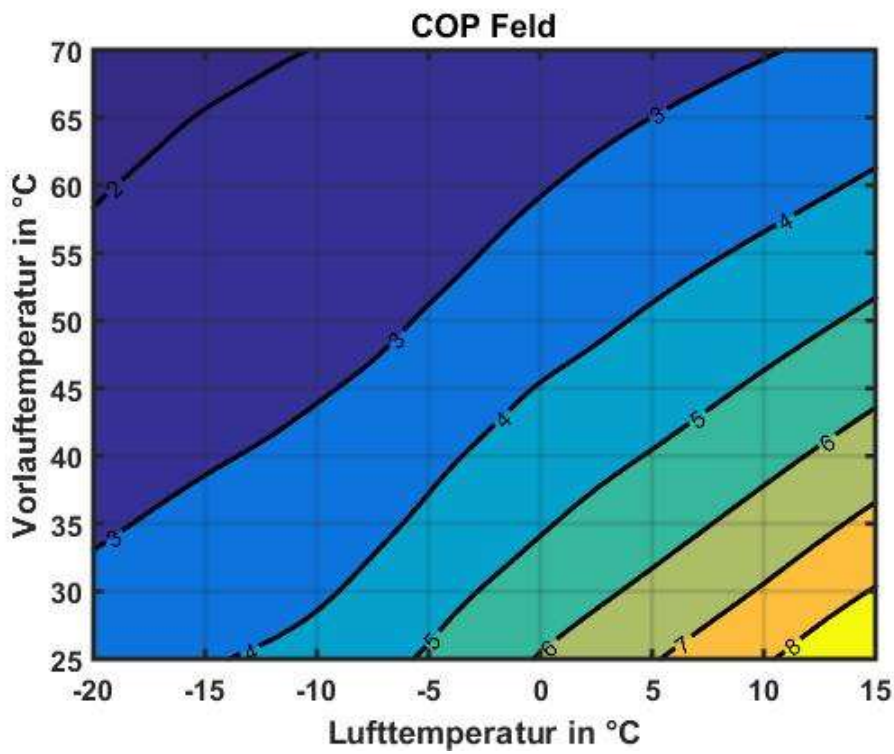
Abbildung 31: EU13L bei 9kW Heizleistung
