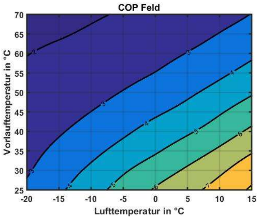
Abbildung 32: EU08L bei 6kW Heizleistung
