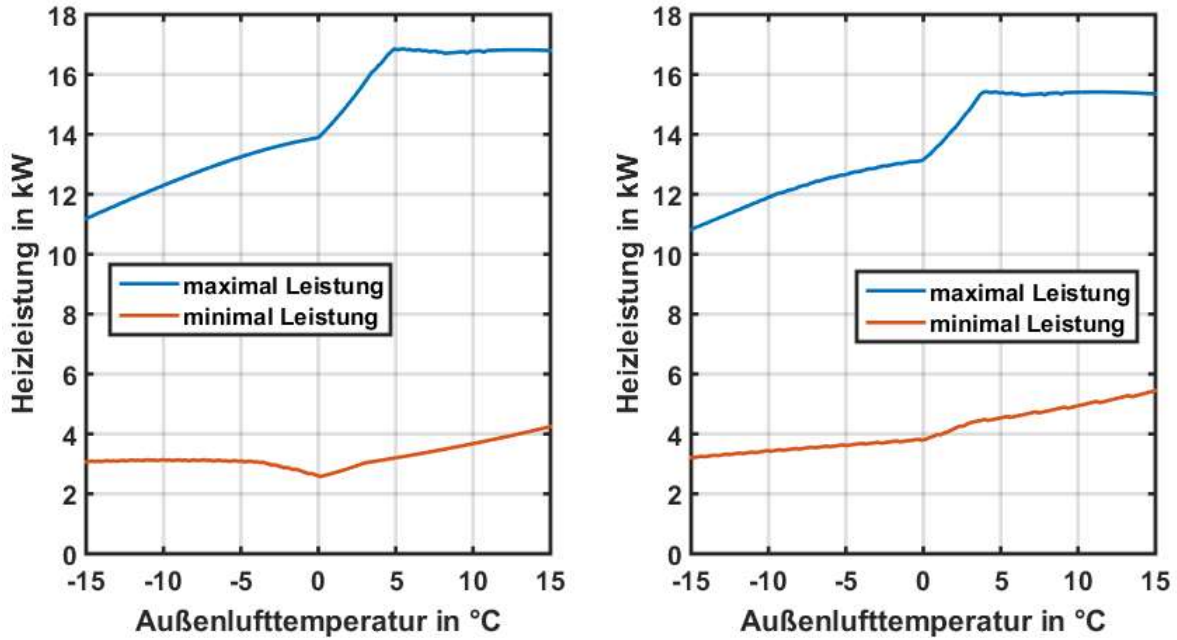
Abbildung 27: EU13L bei 5K Spreizung (links: 35°C Vorlauftemperatur / rechts: 55°C Vorlauftemperatur)
