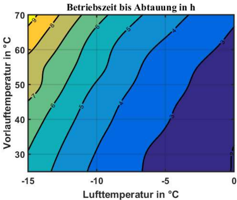
Abbildung 34: Betriebsdauer zwischen Abtauzyklen bei 6kW Heizleistung und 95% Luftfeuchte
