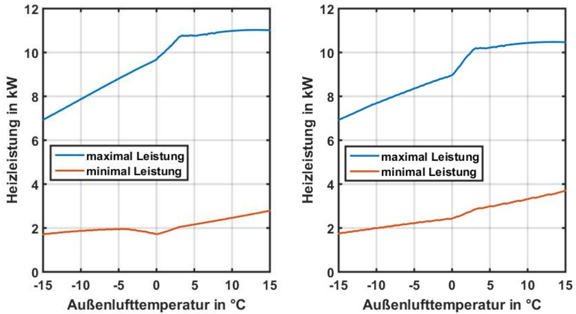
Abbildung 29: EU08L bei 5K Spreizung (links: 35°C Vorlauftemperatur / rechts: 55°C Vorlauftemperatur)
