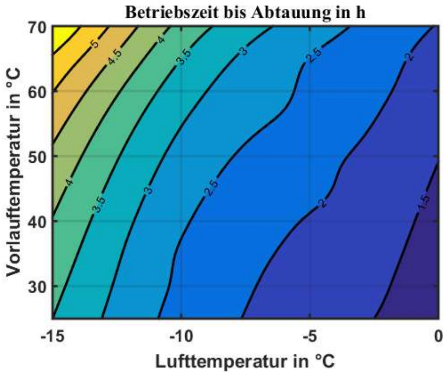
Abbildung 33: Betriebsdauer zwischen Abtauzyklen bei 9kW Heizleistung und 95% Luftfeuchte
